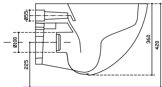
Sezione/ Section/ Section/ Sección
