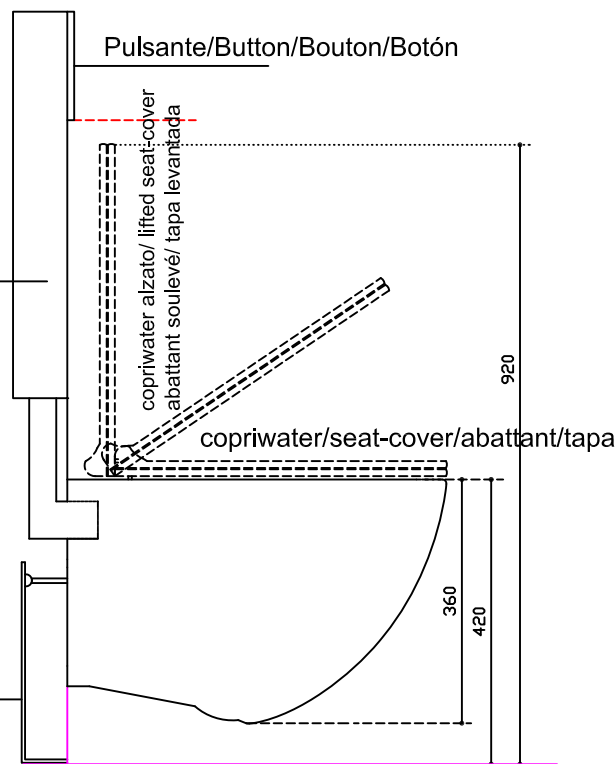
Vista laterale/side view/ Vue latérale/ Vista lateral
