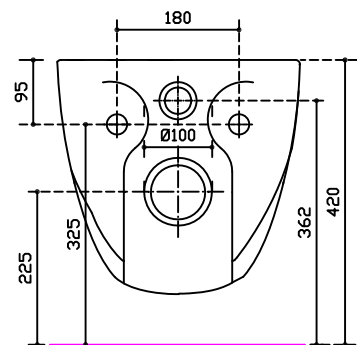
Vista posteriore/ Back view/ Vue arrière/ Vista posterior
